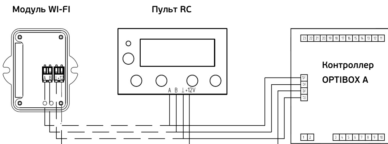
Рис. 2.2 Подключение средств ДУ
