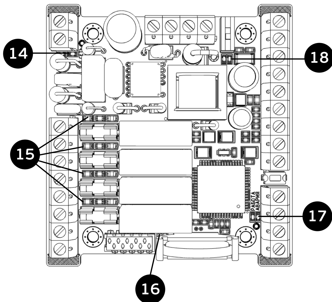
Рис. 1.2. Индикаторы контроллера.
