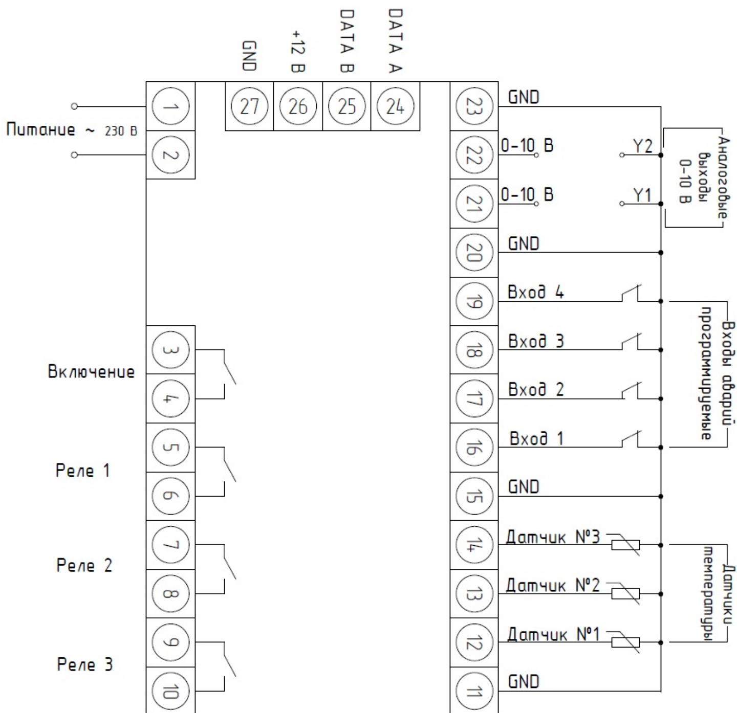
Рис. 2.1 Расположение клемм.
